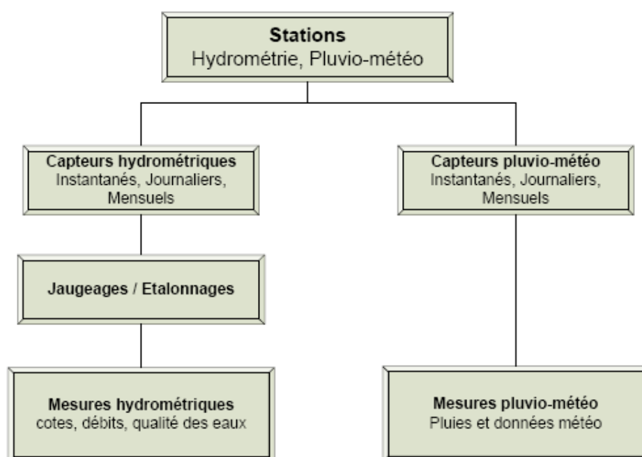
Figure 6 : Structure de la Base de Données « HYDROM » de la DGRE
