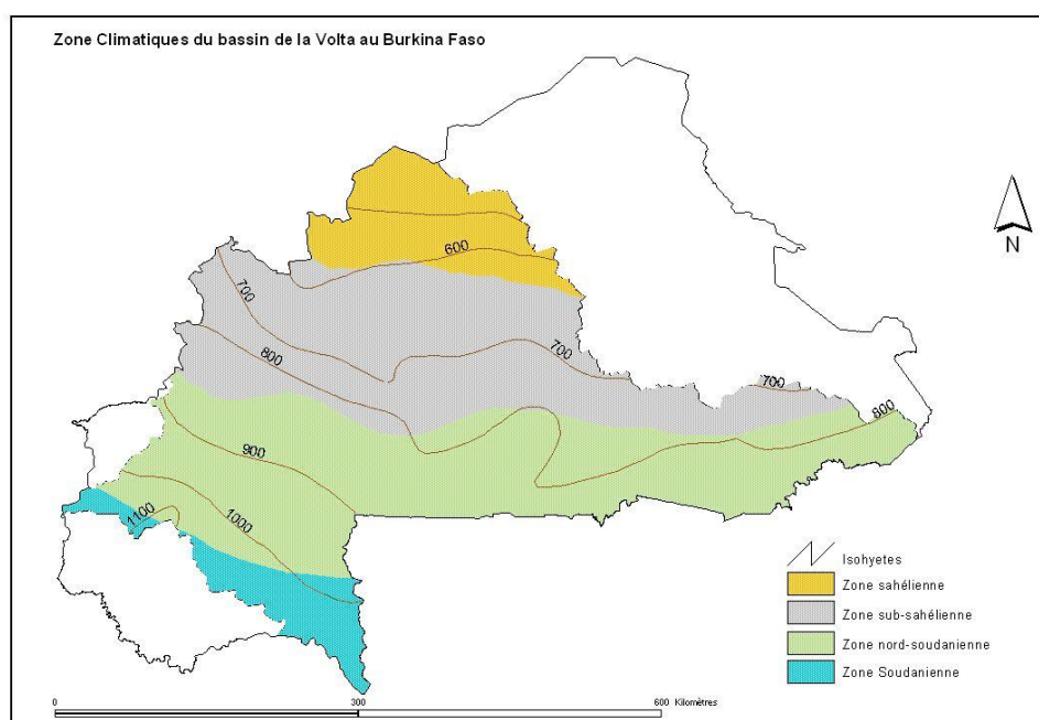
Carte 3 : Zones climatiques du bassin de la volta au Burkina
